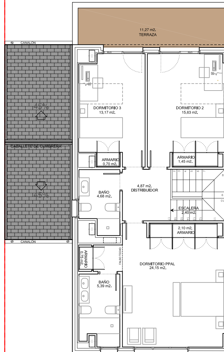
PLANTA PRIMERA
